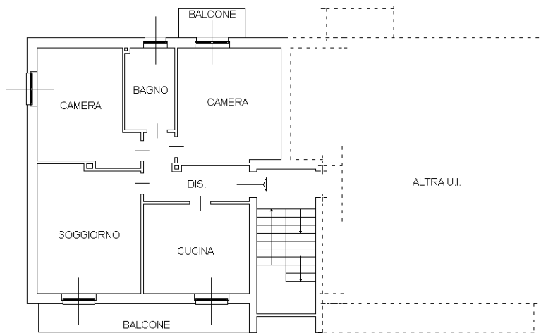
PIANO PRIMO H=3.00 MT
